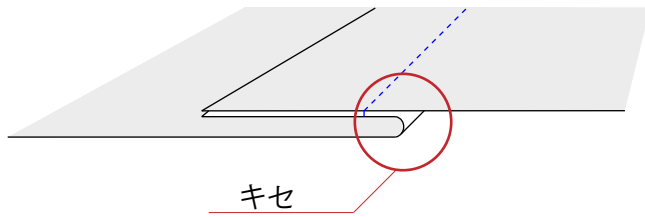
① キセをかける ※キセの深さは通常 5 厘以下
